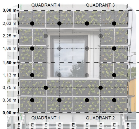
Abbildung 12: Konzeptionelle Darstellung zur Aufnahme des kubischen Pflanzenvolumens an der wandgebundenen Vertikalbegrünungsvariante mit Fensterausparung (IBLB, BOKU University, 2024).
