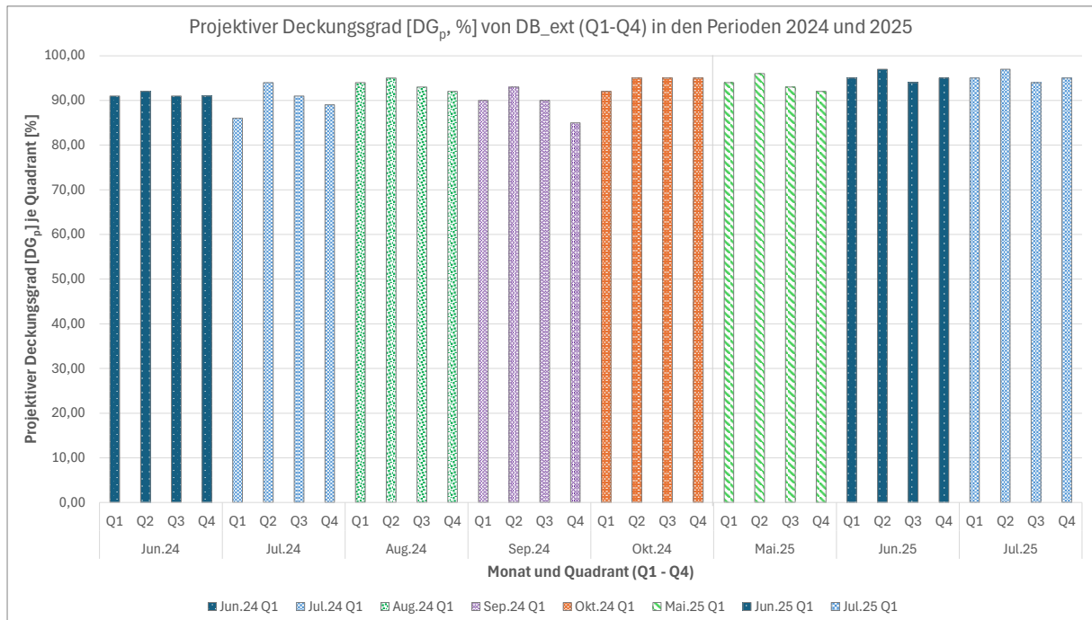
Abbildung 59: Entwicklung von DG p [%] am Gründachteststand je Quadrant (Q1-Q4) in den Vegetationsperioden 2024 und 2025 (IBLB, BOKU University, 2025).
