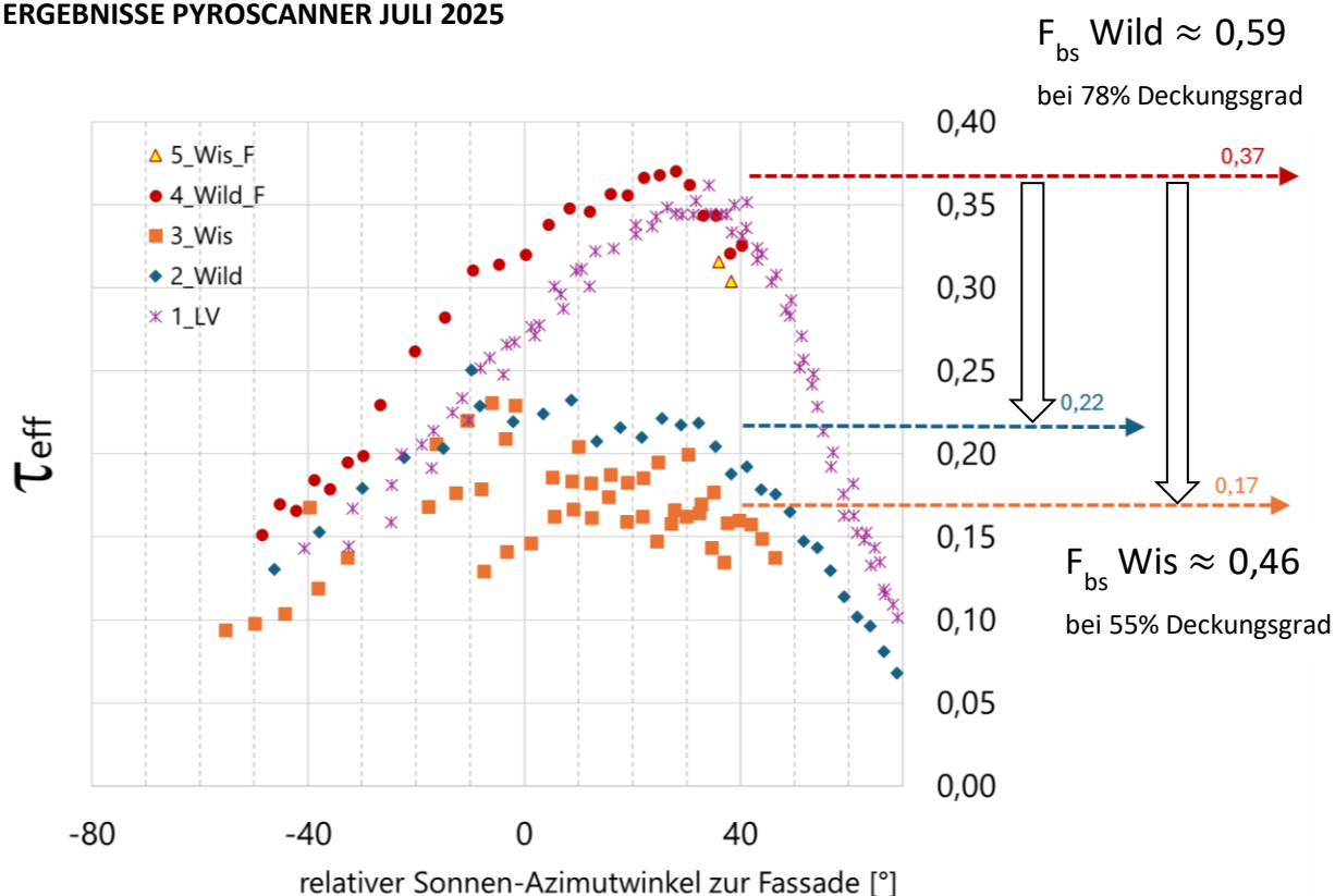
Abbildung 47: Messzeitraum Juni/Juli 2025. Messung des effektiven Transmissionsgrades durch die Verglasung mittels Pyroscanner und Umrechnung in den Bioshading coefficient F_{\text{bs}} . Es wurden nur Messpunkte mit Diffusstrahlungsanteil unter 50% berücksichtigt.
