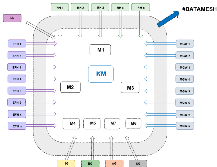
Abbildung 1: Datenraum für das Monitoring von Gebäuden
