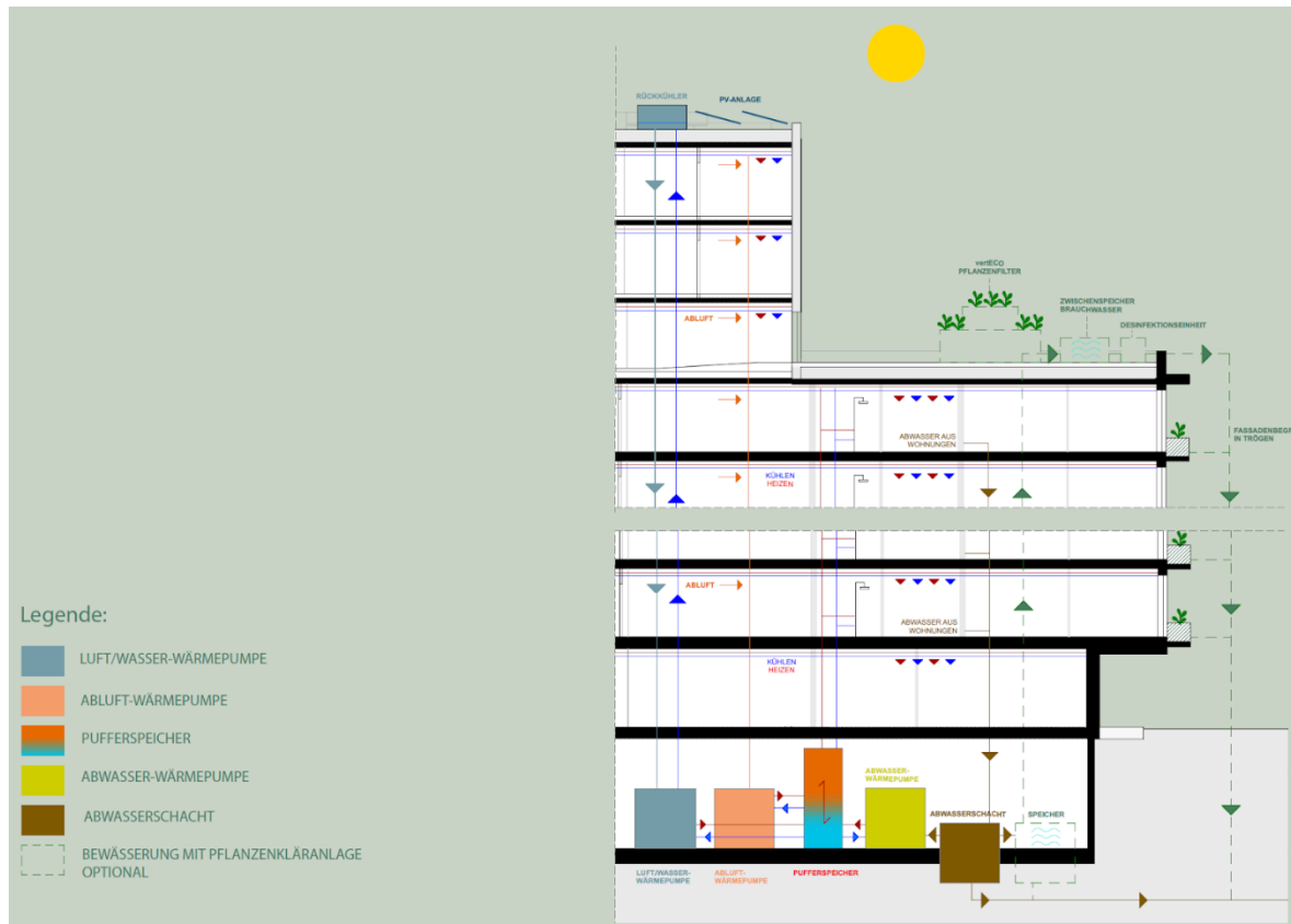
Abbildung: FavoriteFlows
