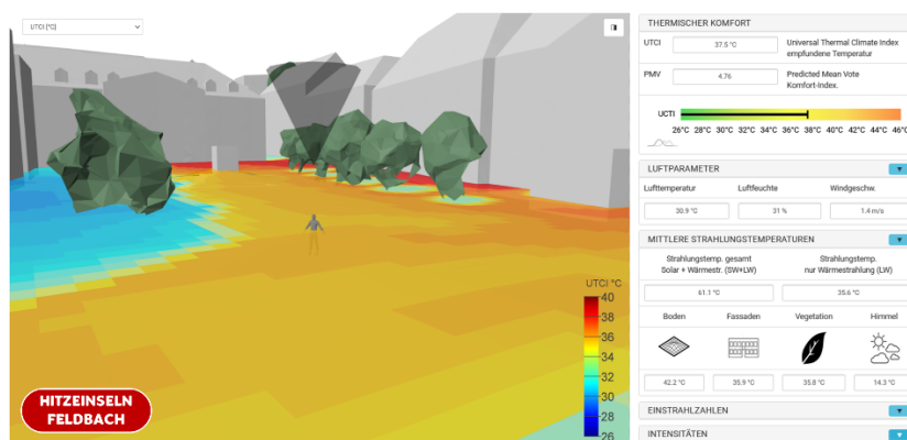
Abbildung 3: Sampling
