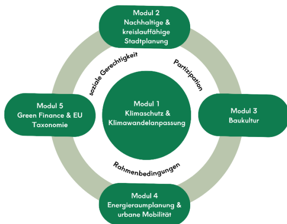
Abbildung 1: Methodik
